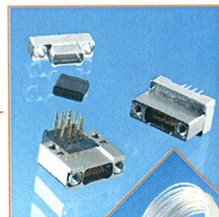
Extreme miniaturisation Nano-D
